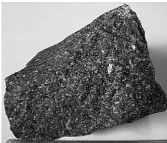
Образец долерита
