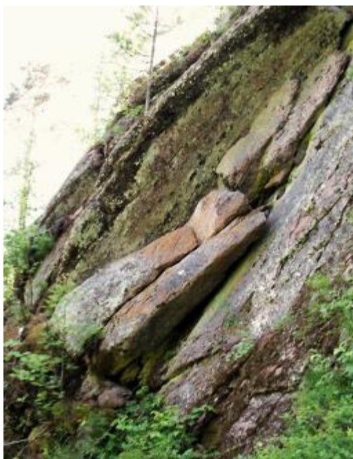
Скалы «Соколиные»
